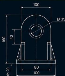
DETALHE AMPLIAÇÃO A ESCALA A2
